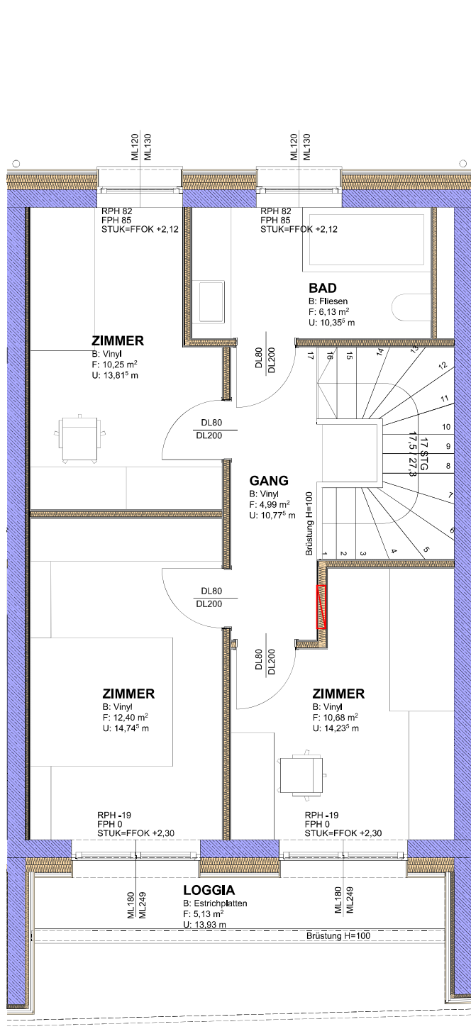
OG
